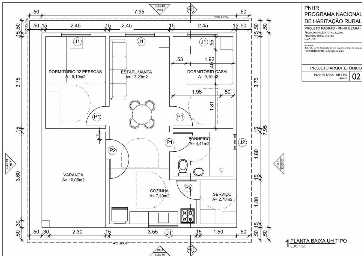
Figura 01. Planta baixa da casa padrão - PNHR.
